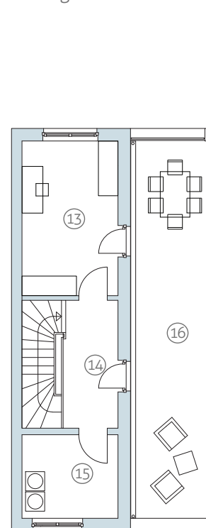
Staffelgeschoss / Penthouse
